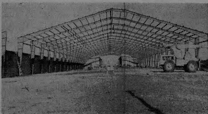
EDIFICIO COTICA, Fábrica de PLYWOOD que en total tendrá un área de 100.000 (cien mil) metros cuadrados. Se han construido hasta la fecha 7,750 m 2 y tenemos en construcción 2,500 m 2 más.
